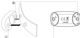
取付方向図
